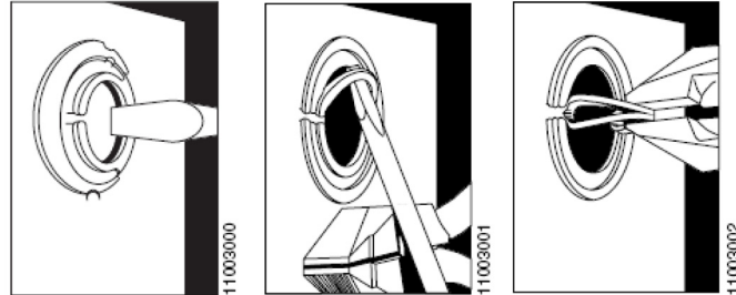
TABL. 1 : Bolt-on Conduit Hubs / Receptáculos para tubo conduit atornillables / Manchons de conduit à boulonner Figure / Figura / Figure 1 : Removing Knockouts / Extracción de los discos desprendibles / Retrait des débouchures
