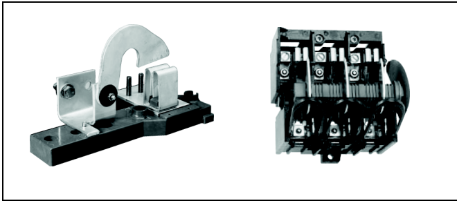
FIG. 3 : Examples of Line Base Assemblies / Ejemplos de ensambles de la base de línea / Exemples d'assemblages de la base de ligne
