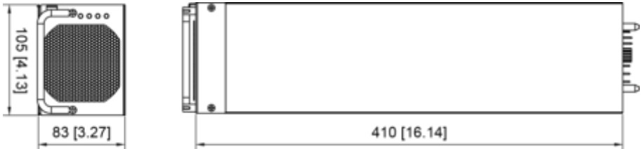
Schéma 1. SR-1600 Plus – Encombrement onduleur
